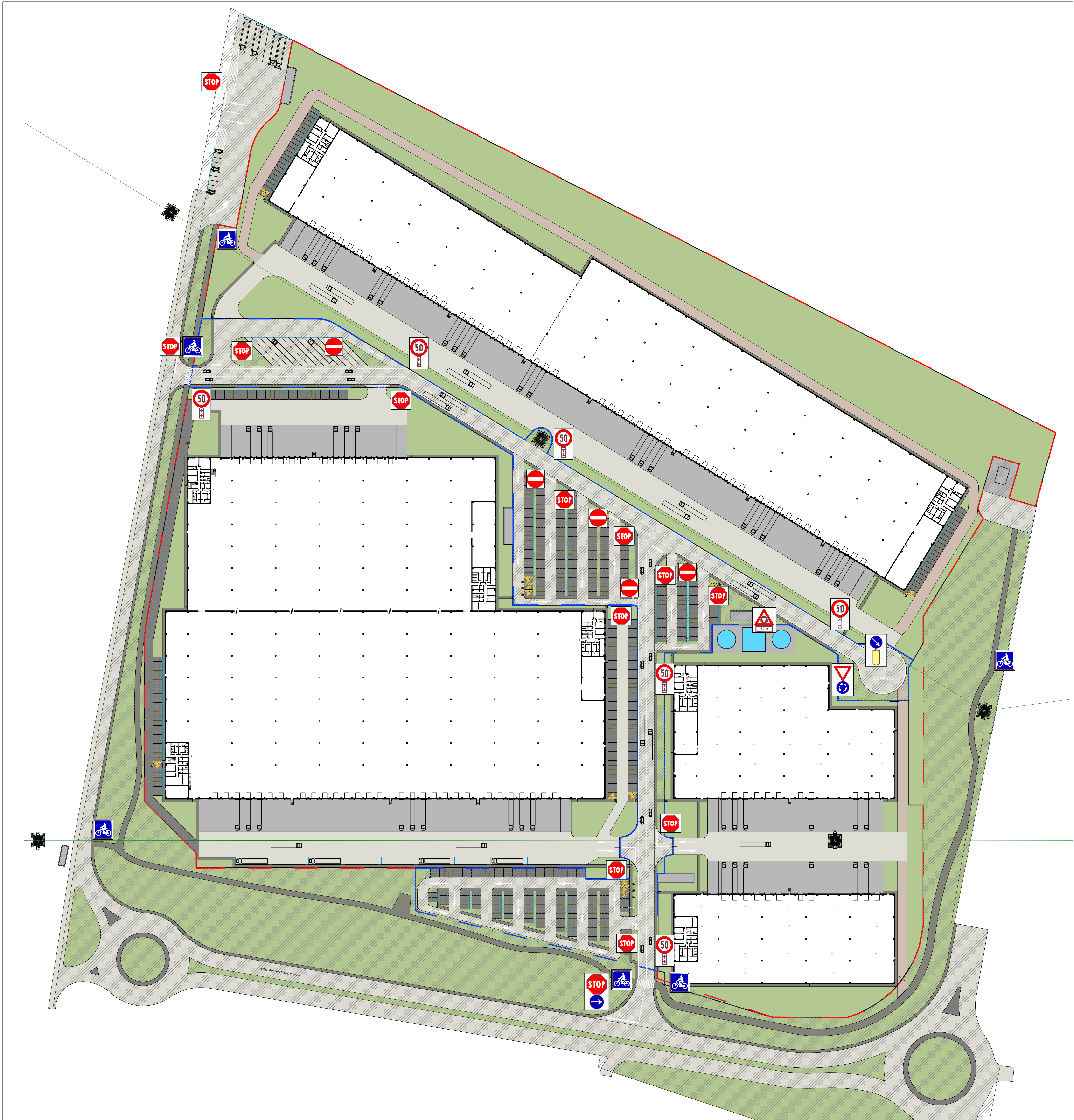
TAVOLA VIABILITA' Scala 1 : 1.000
